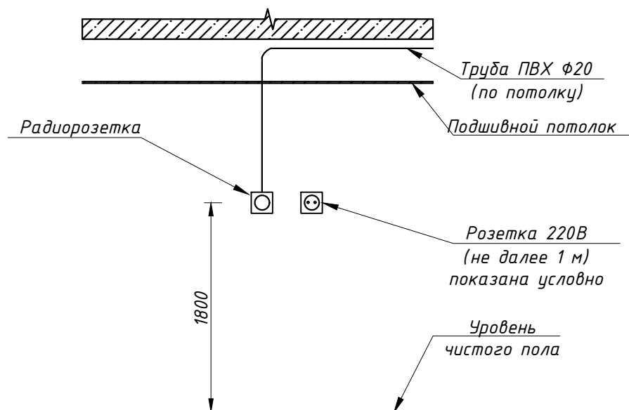
Узел 1 М 1:50
